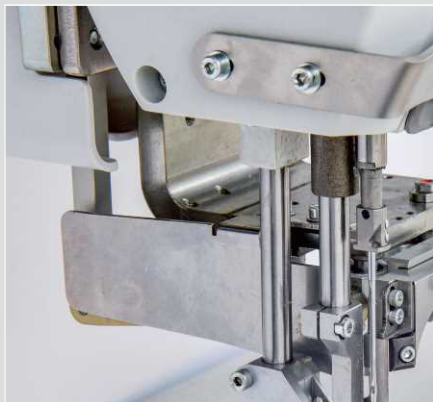
独立电机驱动的垂直式切边装置
