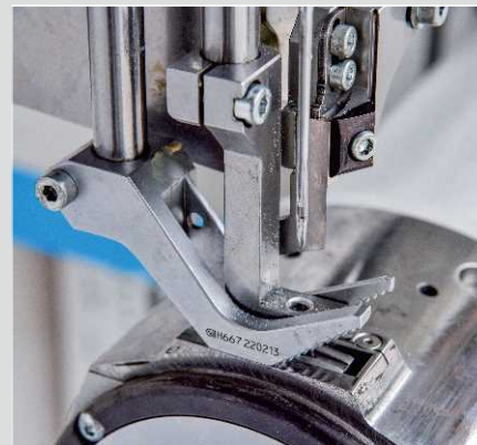
XL筒型摆梭设计，锁芯容量增加70%
